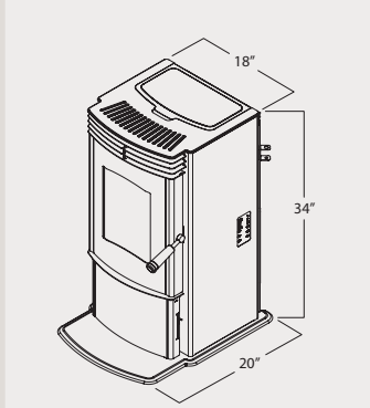
Mini Pellet Stove
